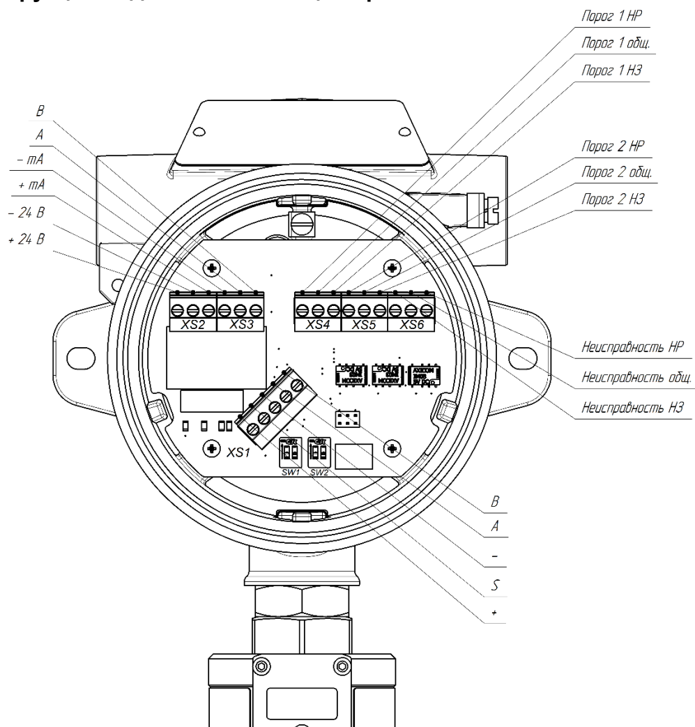
Рисунок 4.2 – Чертеж подключения с опцией реле
